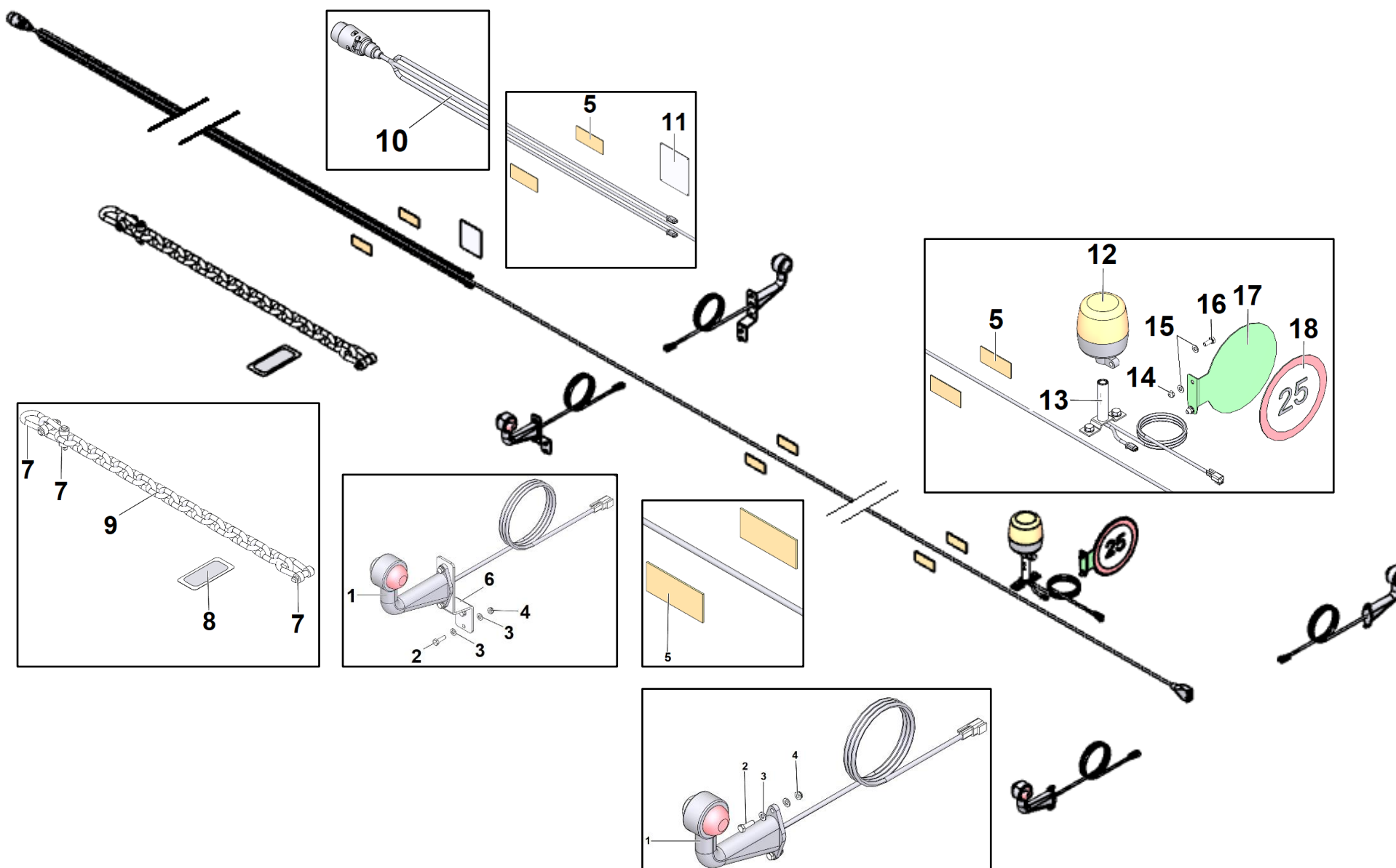
TAVOLA 12 - TABLE 12 - PLANCHE 12 - DISEÑO 12 KIT OMOLOGAZIONE FRANCIA
